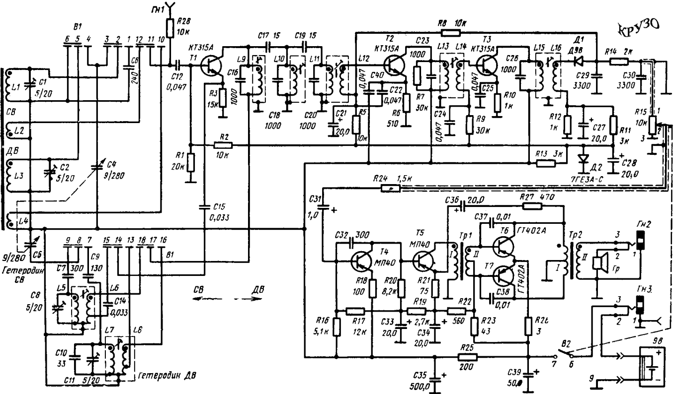
Принципиальная электрическая схема радиоприемника «Альпинист-407»
